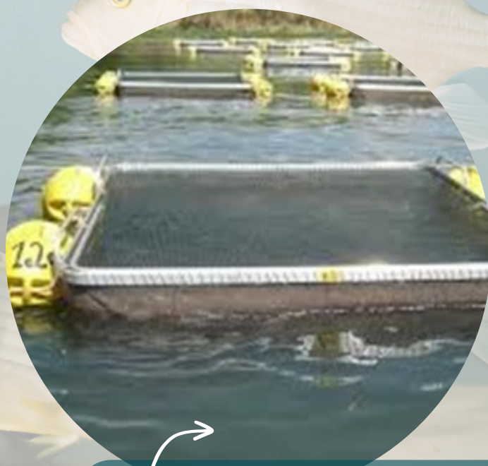
BMDNET AQ Tanque rede com bolsão em formato quadrado
